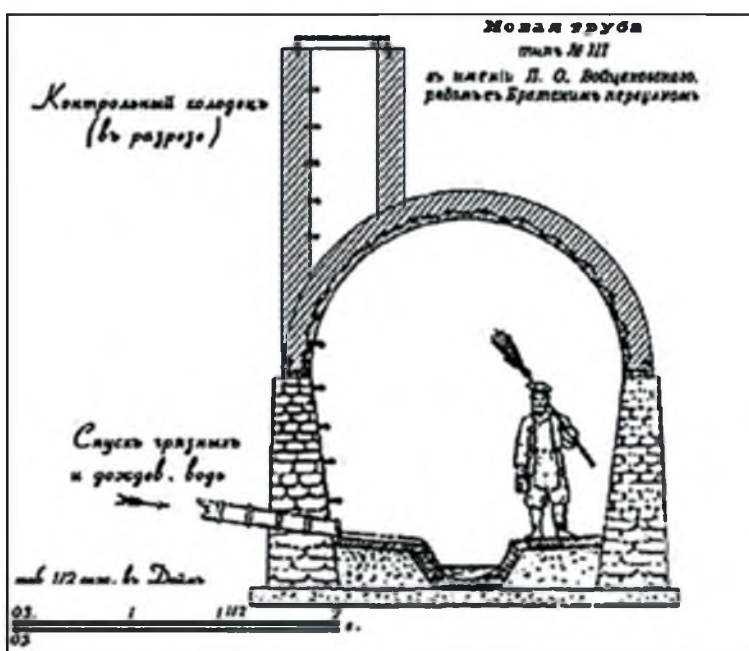
Рисунок 4. Генеральный коллектор в разрезе. Рисунок конца XIX в.
