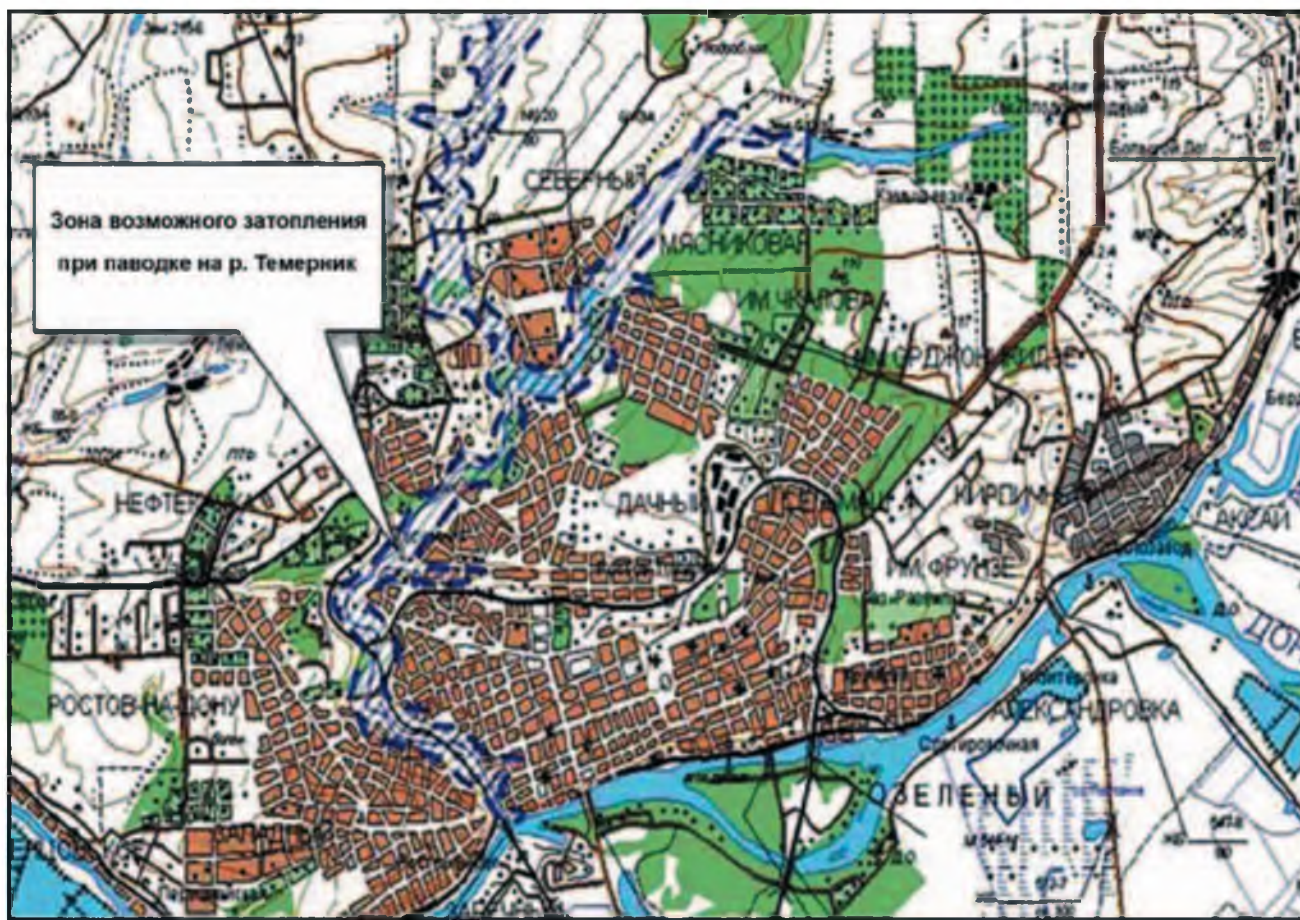
Схема 3. Зона возможных затоплений при паводках на реке и балке Темерник
