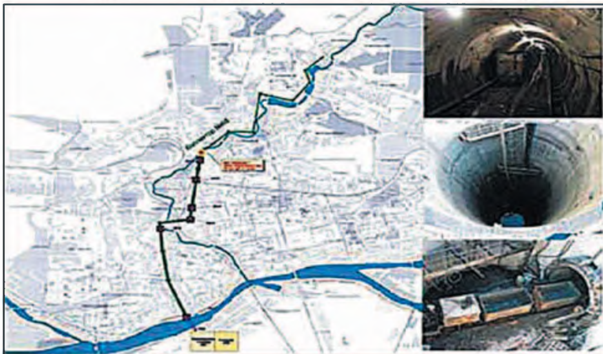
Схема 5. Трасса подземного канализационного коллектора №68
